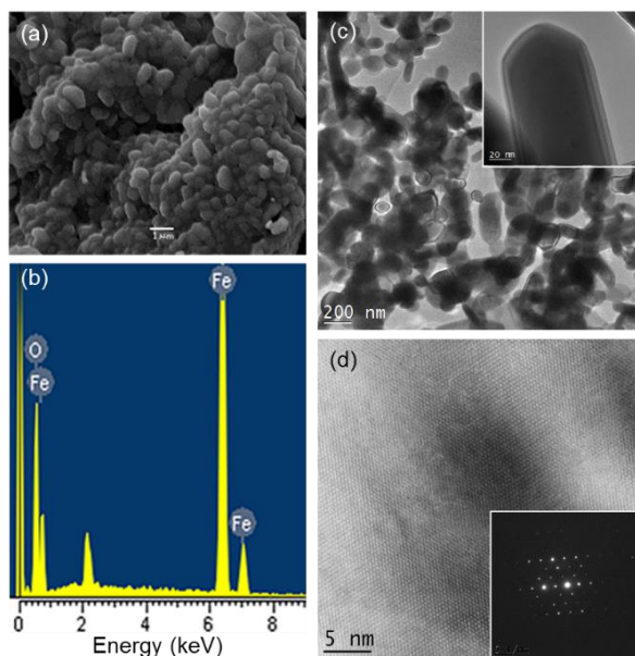
Fig. 5. (a) SEM, (b) EDS, (c) TEM, and (d) HRTEM analysis of the pyrolytic crystalline materials from 1:1 Chitosan•(FeCl 3 ) y precursors. Contrast in (d) arises from thickness variations.
