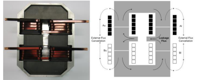
Fig. 2. CCTT IM coupled inductor.
