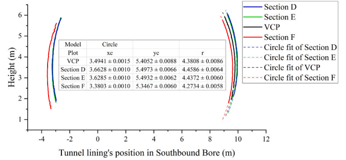
(d) Layby tunnels cross section comparison in SB
