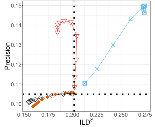
(d) Prec./ILD S trade-off on TastePro- file
