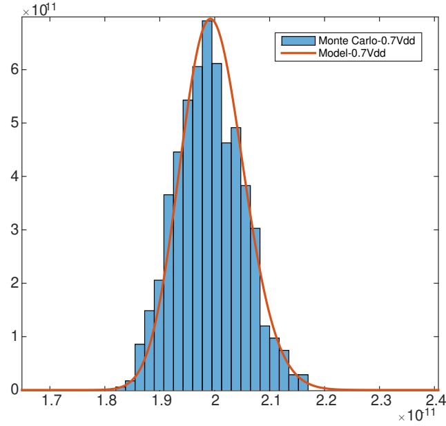
(b) V_{dd} = 0.7 \text{ V}
