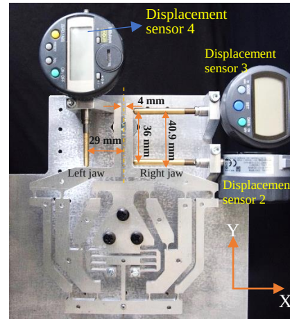
(d) Set-up for testing the jaw performance
