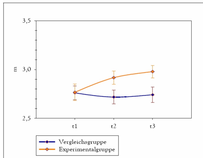
Abbildung 3: Mittelwerte (m) und Standardabweichungen (s) bei Experimental- und Vergleichsgruppe für die Messzeitpunkte t1, t2, t3 für die Skala „Offenheit und Aufgeschlossenheit“ (Wertebereich: 1,0 bis 4,0)
