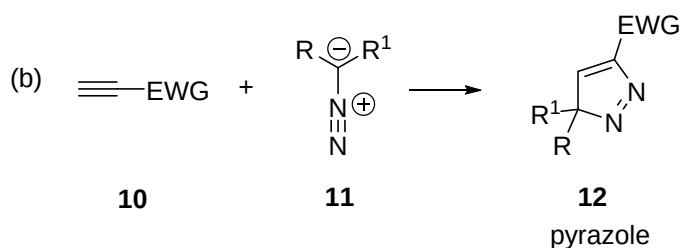
Scheme 1.4
