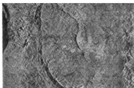
ESTAMPA 3 Folha SB.22-Z-B — Imagem de radar, escala 1:250.000 — Anticlinal elevado do Rio Lombo, Folha de Xambioá. Observa-se no centro, um traço antecidental acentuado por perfilamento. As estruturas alinhadas pela areia formam “hog back”. À direita, a borda da Bacia Sedimentar do Piau-Mesquita. À esquerda, margem do Rio Araguaia. Os terrenos elevados pertencem ao Pediplano Piauíocênico. O Rio Lombo está superimposto ao “hog back”.
