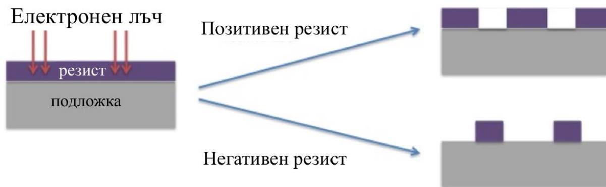
Фигура 1. Схематично представяне на процеса на електронна литография.
