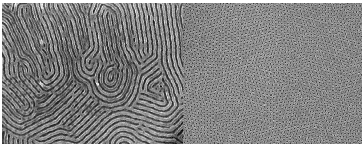
Фигура 2. Две спонтанни BCP изображения, снимани със сканиращ електронен микроскоп (СЕМ) – едното наподобяващо пръстов отпечатък, а другото във формата на вертикални цилиндри. Размерът на линиите и точките на двете снимки е около 20 нм.
