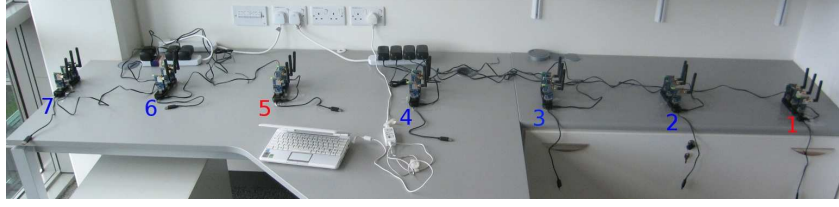
Fig. 18. Testbed
