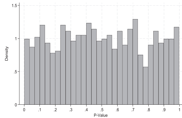
(d) Out-of-Sample Permutation – P-Value
