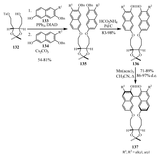
Scheme 25.
