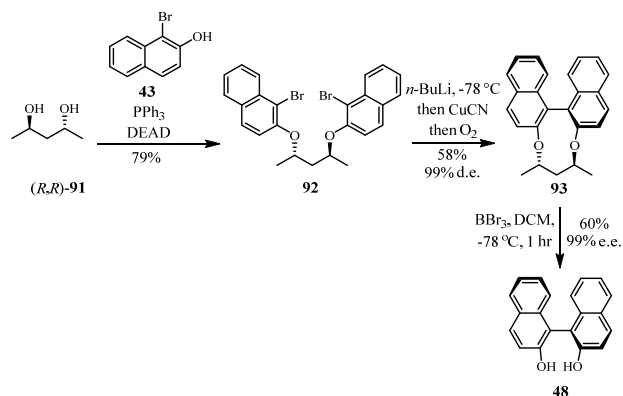
Scheme 16.
