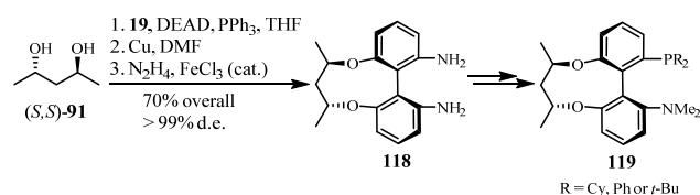
Scheme 22.
